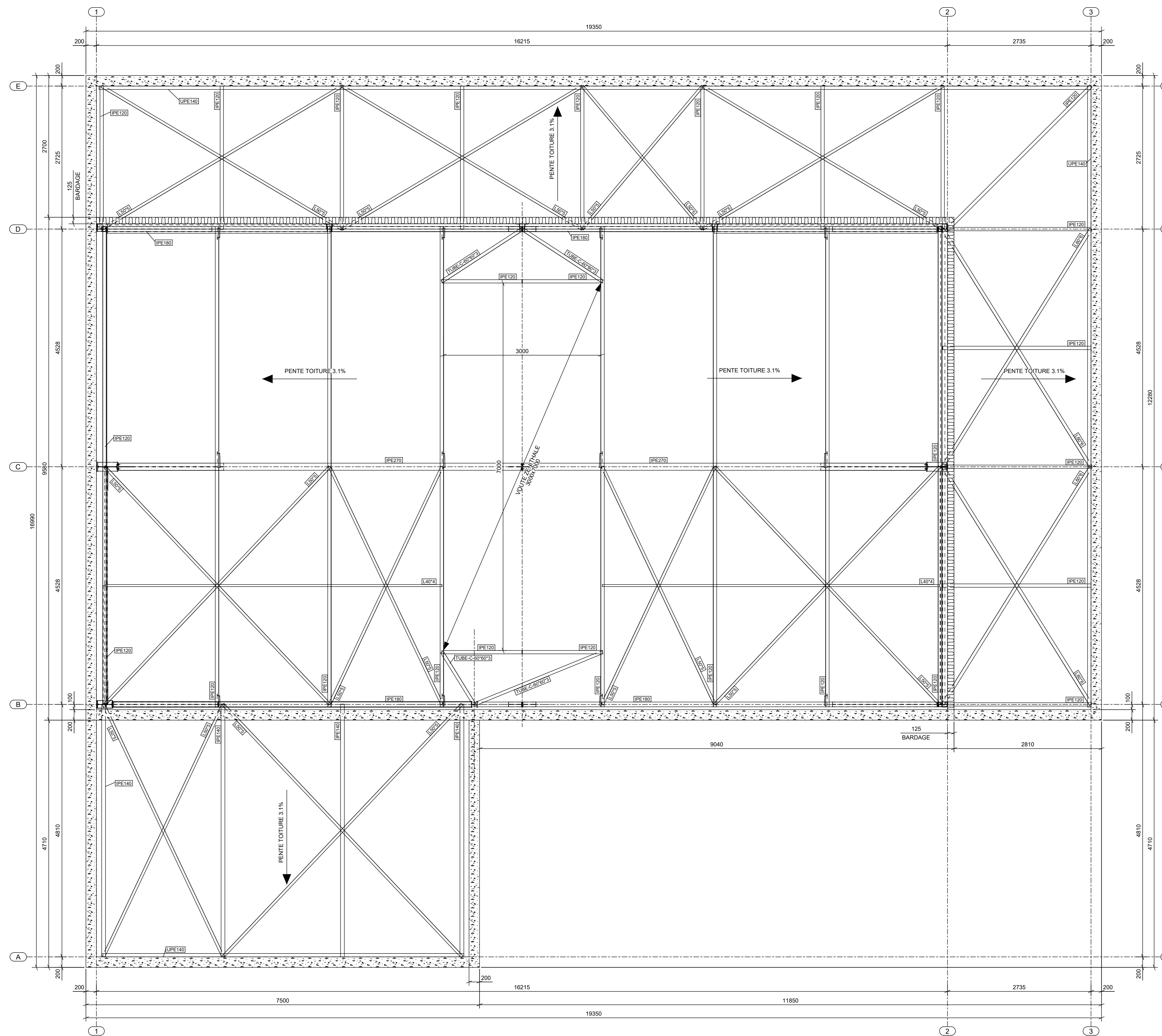
TOITURE 1:33
